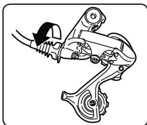
Obr. 6 Nastavovací matica pri zadnom preadačovači. Obr. 6 Nastavovací matice měniče převodů.
