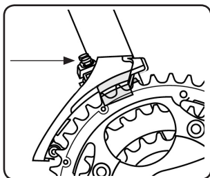
Obr. 7 Nastavovacie skrutky predného preadačovača. Obr. 7 Šrouby nastavení dorazů přesmykače.
