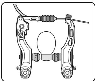
Obr. 8 Ráfiková brzda typu „V“. Obr. 8 Ráfková brzda typu „V“.
